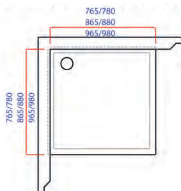
Inbouw maat douchebak bovenzijde gelijk met vloertegels
