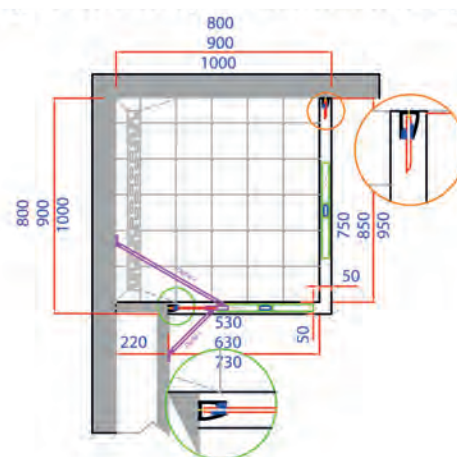
Dorpel verwerkt in vloer tegen kolom optie stabilisatiebeugel
