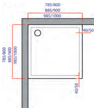
Inbouw maat douchebak boven op de vloer
