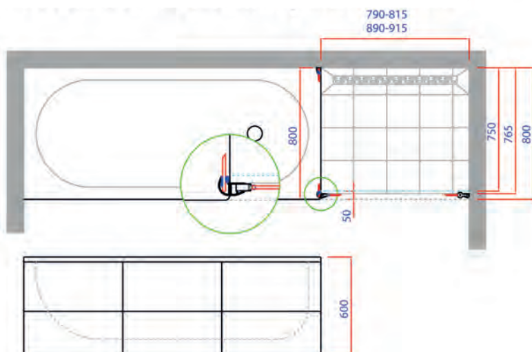
Douchedeur met verkorte zijwand op het bad
