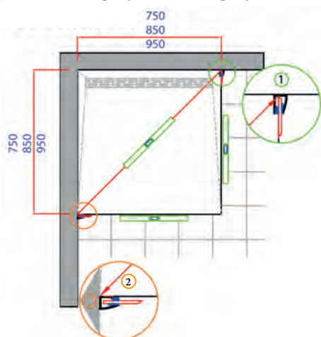
Douchedeur met verkorte zijwand op het bad
