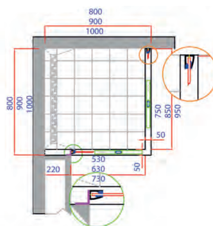
Dorpel verwerkt in vloer tegen kolom optie stabilisatiebeugel
