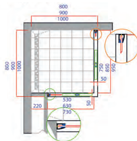
Dorpel verwerkt in vloer langs kolom
