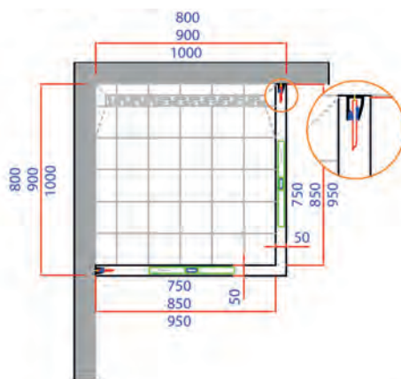
Douchedeur met verkorte zijwand op het bad
