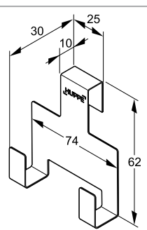
Houder voor wisser
