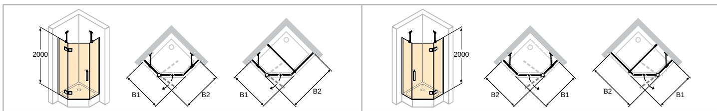
Bevestiging links Breedte zijdeel vanaf 600mm met dwarsbeugel
